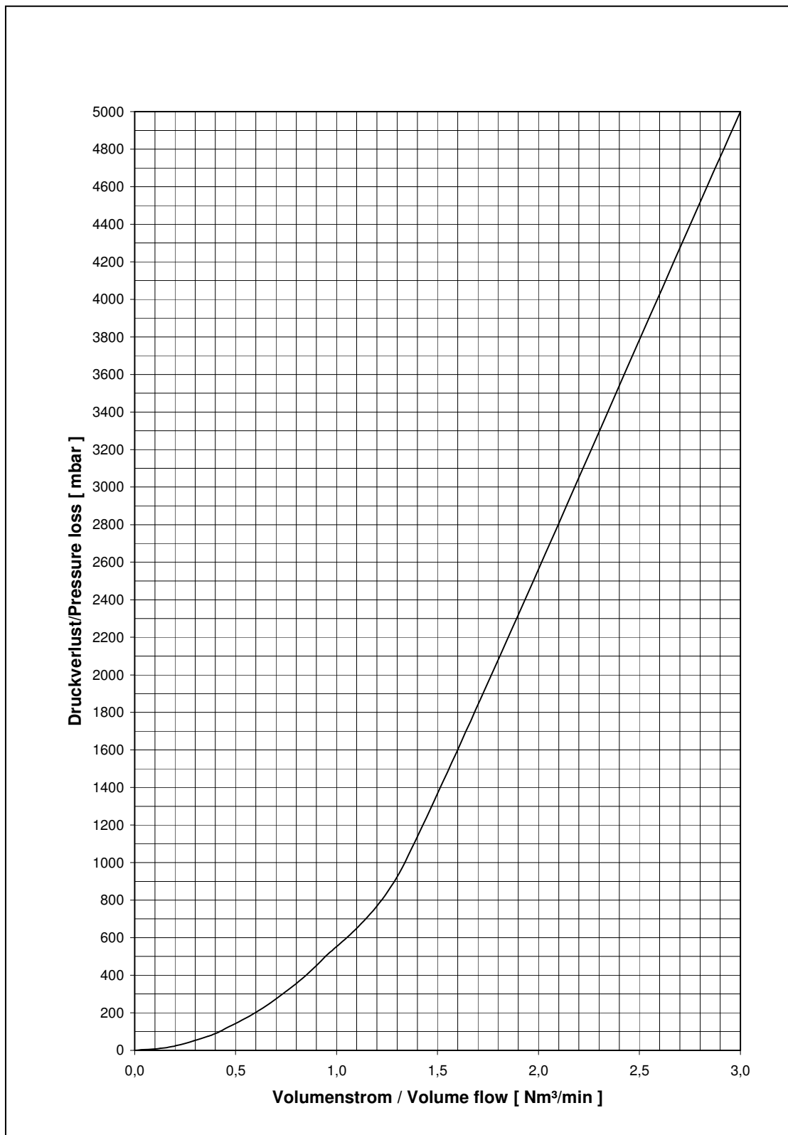
Bild 2 Druckverlust Medium: Wasser, \rho = 1000 \text{ kg/m}^3 , t = 15^\circ\text{C}
